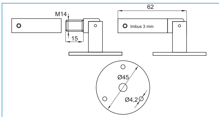
Dolny element mocujący z gwintem M14 do regulacji napięcia linki
