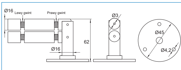
Dolny element mocujący z regulacją napięcia linki
