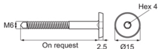
ŚRUBA Z ŁBEM PŁASKIM
