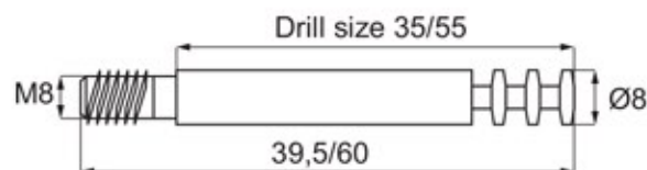
TRZPIEŃ M8
