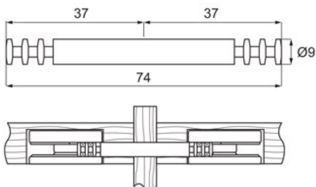
TRZPIEŃ PODWÓJNY
