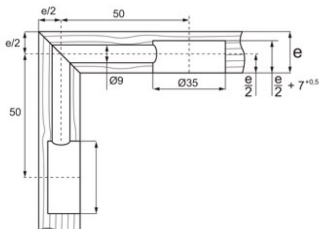
TRZPIEŃ 90 STOPNI
