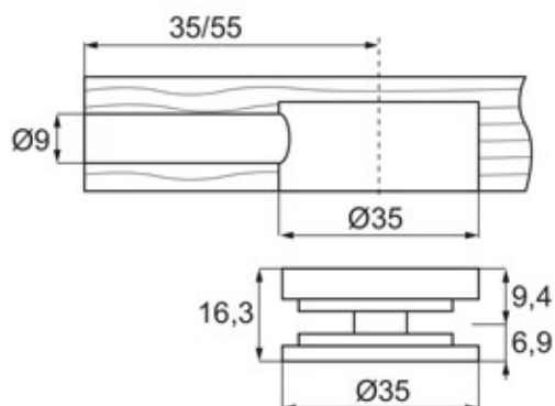
MIMOŚRÓD FI35
