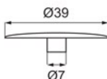
ZAŚLEPKA
