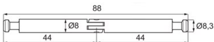
TRZPIEŃ PRZEGUBOWY
