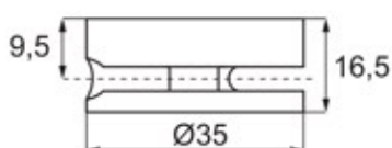
MIMOŚRÓD FI35
