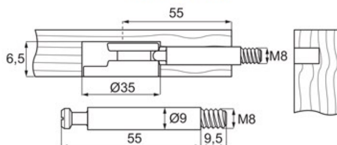
TRZPIEŃ M8
