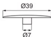
ZAŚLEPKA
